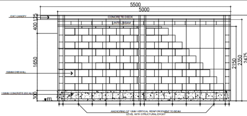
1 LONGITUDINAL ELEVATION S-01 SCALE 1:40
