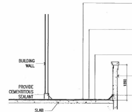
SECTION 2 ROOFDECK W-03 SCALE 1:50 M
